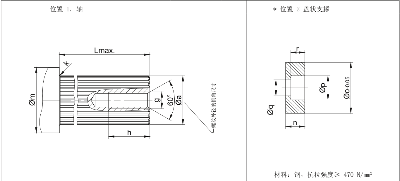
带花键轴的平行轴减速电机安装工具
