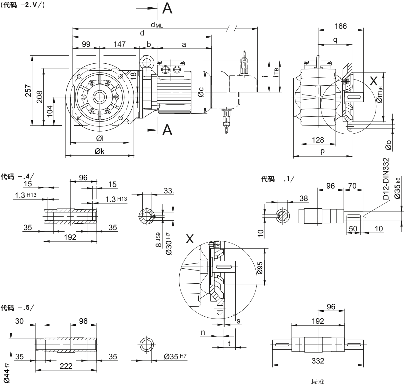
法兰尺寸
