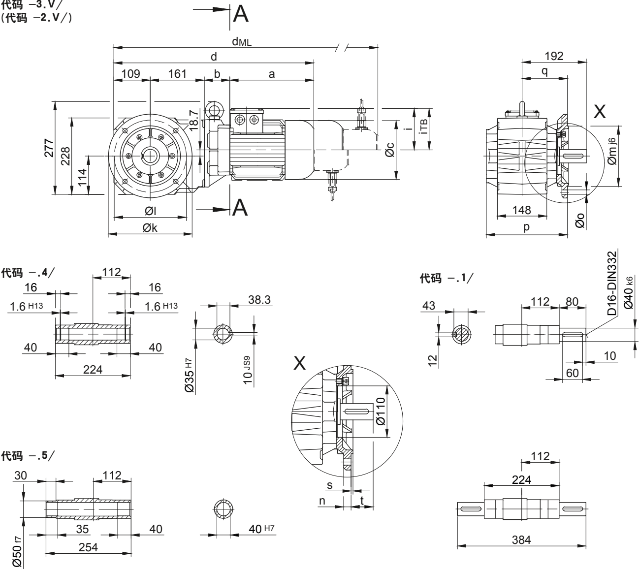
法兰尺寸
