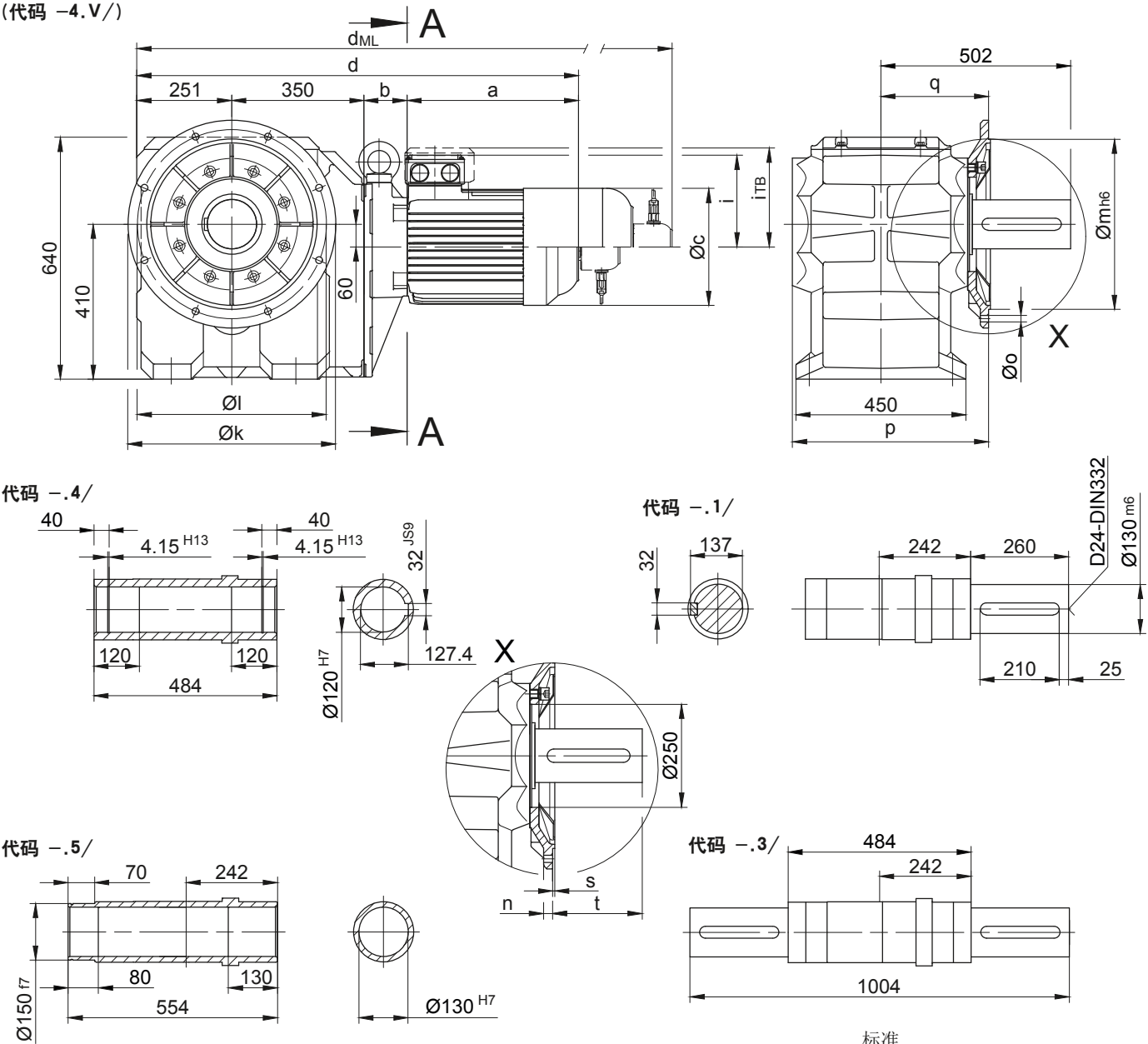
法兰尺寸
