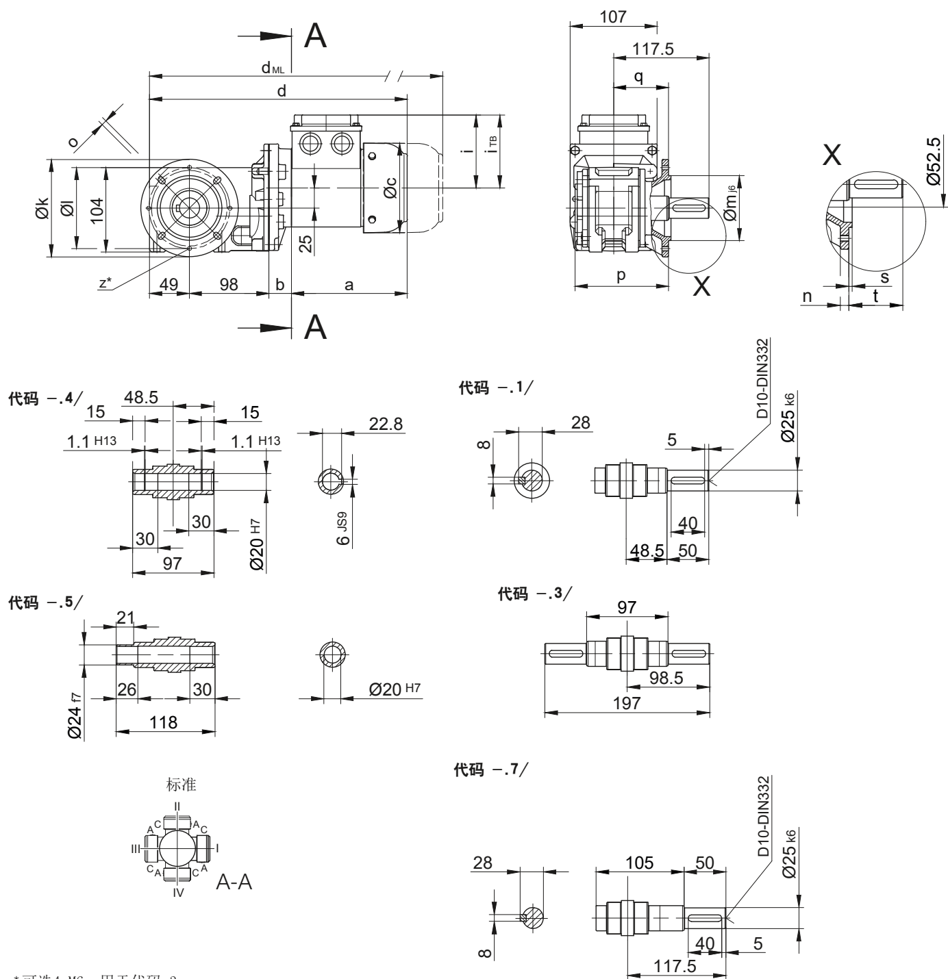
法兰尺寸
