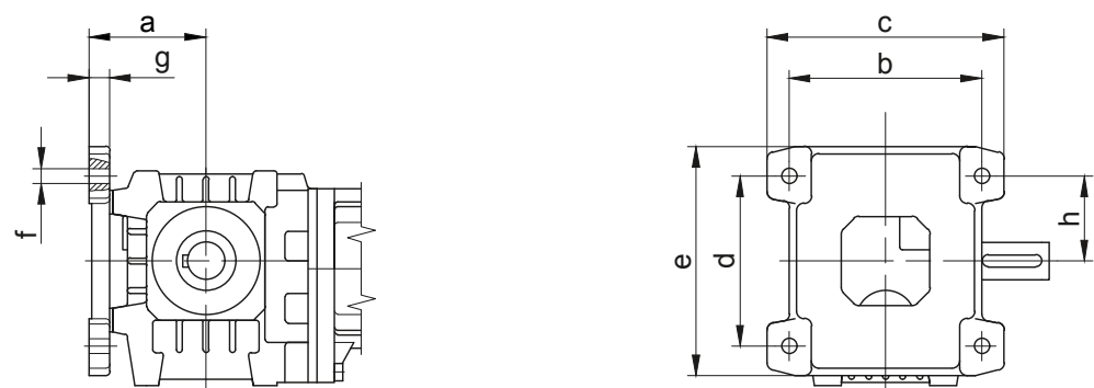
地脚盘，左侧
