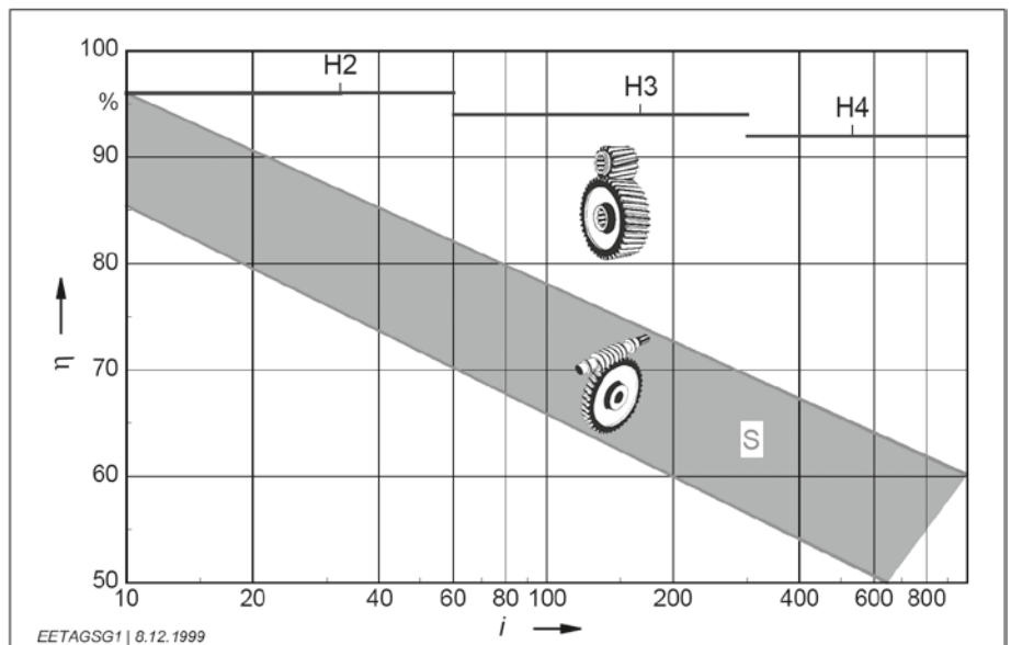
Richtwerte für den Wirkungsgrad ( \eta ) von schrägverzahnten Stirnrad-Getrieben (H) mit 2, 3 oder 4 Stufen im Vergleich zu Schnecken-Getrieben (S) abhängig von der Übersetzung ( i ), bezogen auf Bemessungsleistung des Getriebes.
