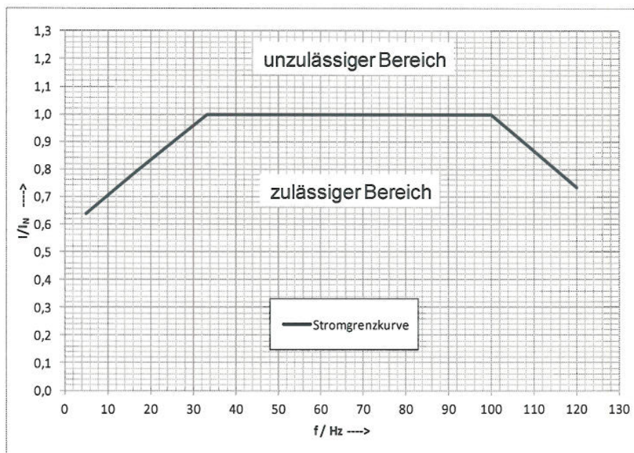
Einstellparameter für die Dauerstromgrenze des Frequenzumrichters zwischen 5 Hz und 120 Hz
