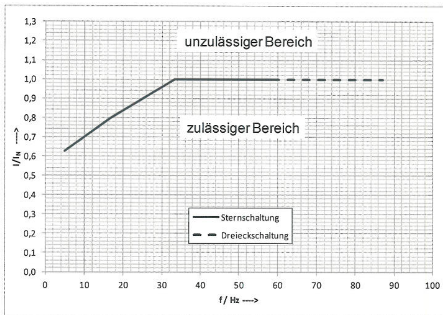
Einstellparameter für die Dauerstromgrenze des Frequenzumrichters zwischen 5 Hz und 87 Hz
