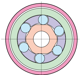
用于双转向与自动换向的超越离合器
